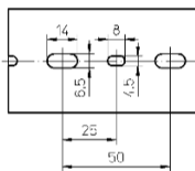
Base punching to DIN 43659
